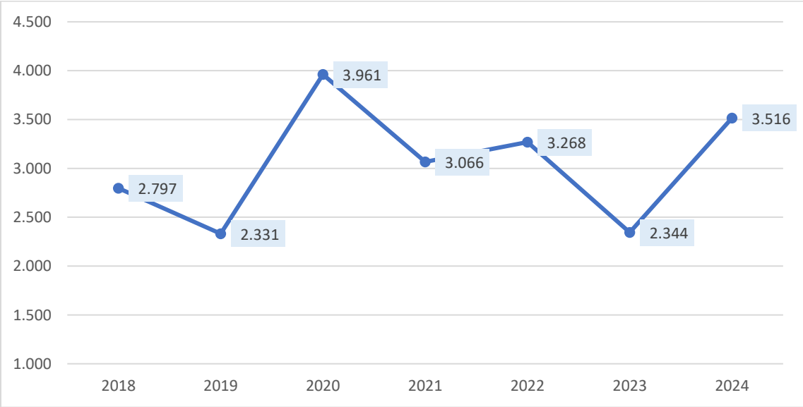
Gambar 2. 3 Tren Curah Hujan Tahunan Kota Balikpapan Tahun 2018 s/d 2024
