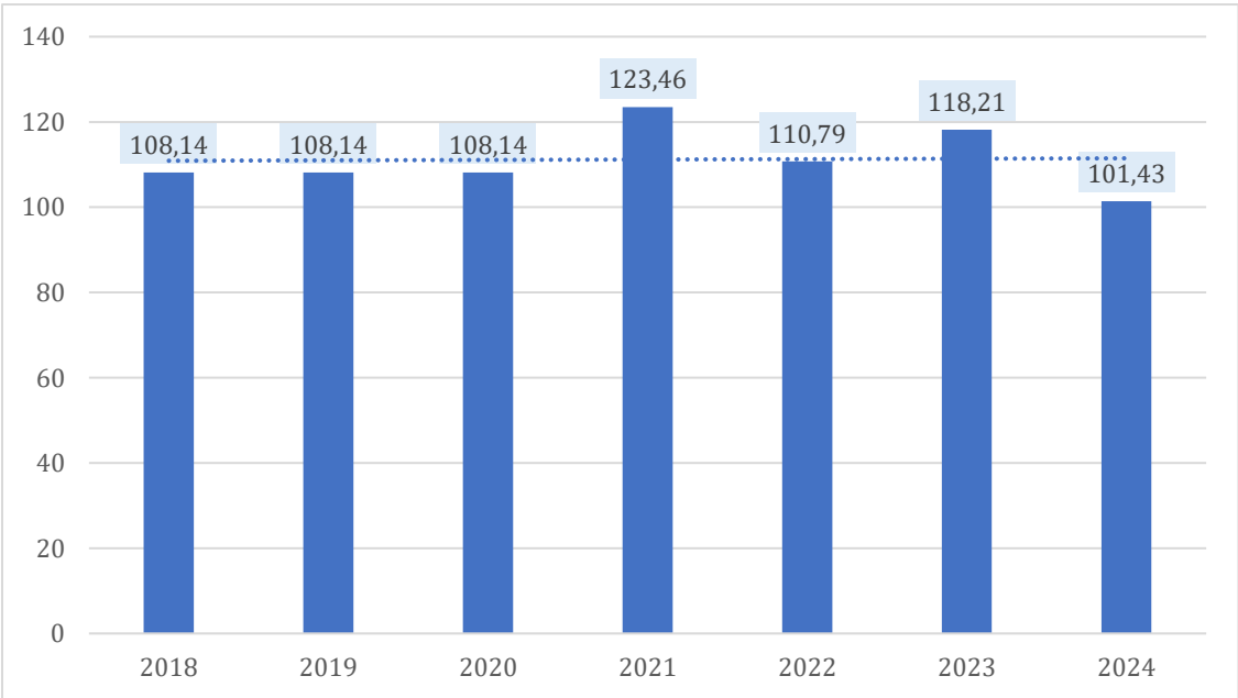
Gambar 2. 4 Indeks Risiko Bencana Kota Balikpapan Tahun 2018-2024
